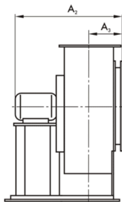
Выходной фланец
