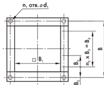
Выходной фланец
