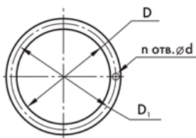
Входной фланец
