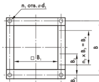
Выходной фланец
