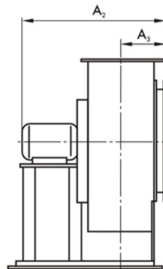
Выходной фланец
