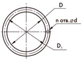
Входной фланец
