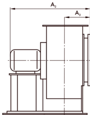
Выходной фланец
