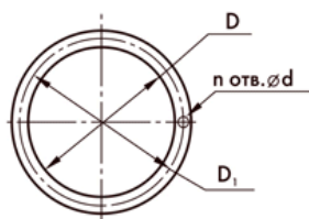
Входной фланец
